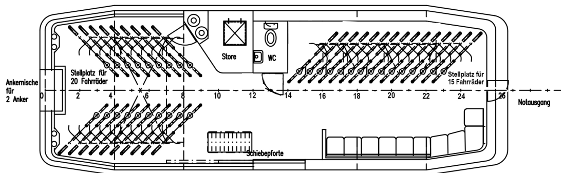
Bodenkonstruktion
